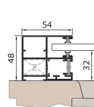
Führungsschiene KR54V
