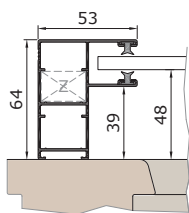
Führungsschiene KD53V
