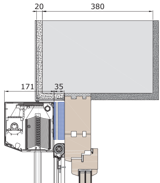
Mit Stockaufdoppelung und Sturzämmung. VORO RAFF (80D) RetroLux mit kombiniertem Insektenschutz-Rollo.
